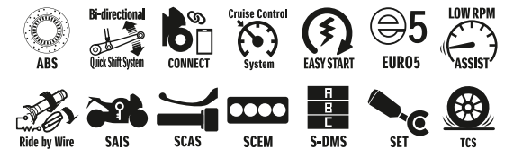
Schwarz (YVB)
