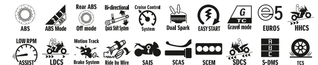
Schwarz (KGL)
