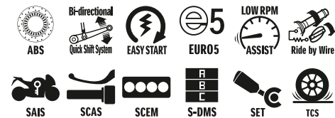
Schwarz (YVB)
