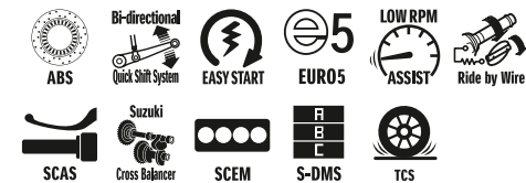
Schwarz (KGL)
